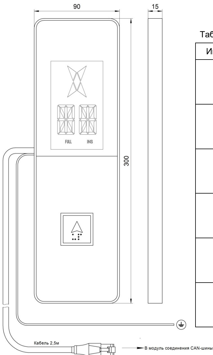
Рис.1 Внешний вид Вызывной пост ОНИКС (жгут RJ45) НШЕК.468381.214
